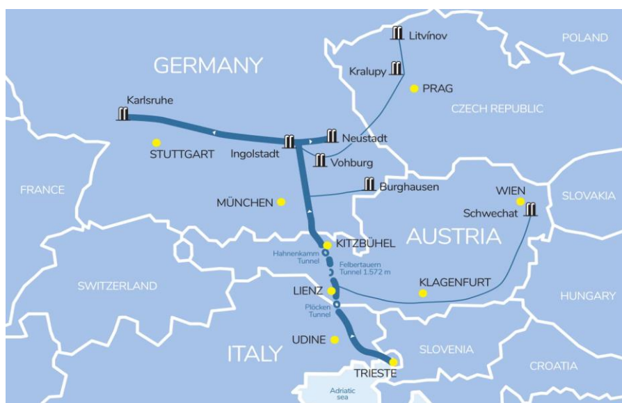
Figura 1 – Oleodotto Transalpino, tracciato
