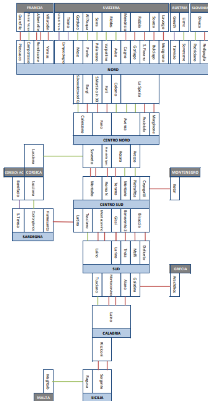
Figura 72: Schema delle linee di connessione fra zone [Fonte: Terna, Individuazione zone della rete rilevante, Allegato A.24 al codice di rete, rev. 05, gennaio 2021]
