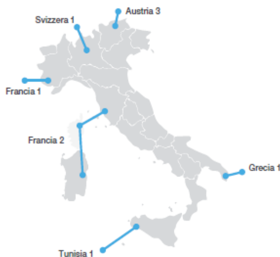
Figura 69 - Progetti di interconnessione pianificati da Terna [Fonte: Terna - Piano di Sviluppo 2023]
