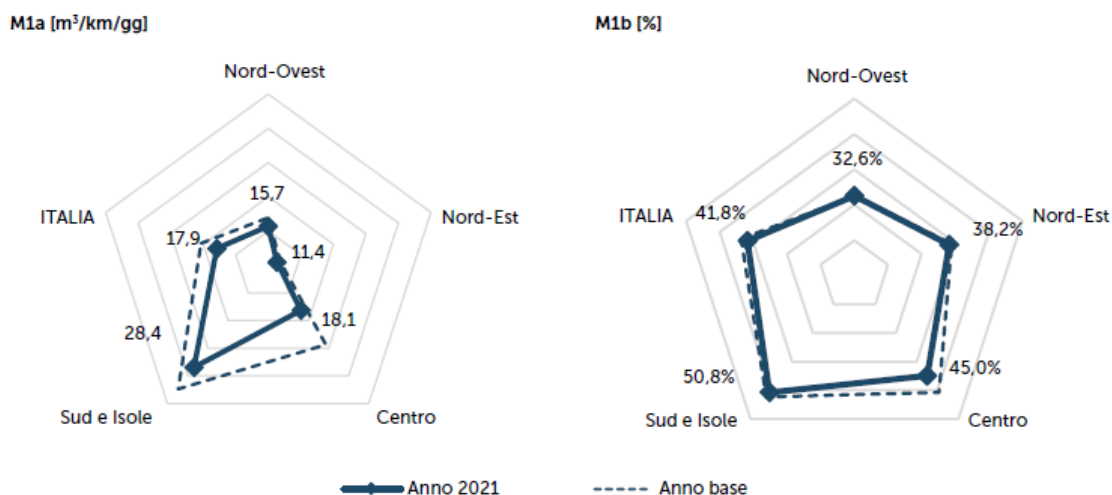
FIGURA 3.2 | Valori medi di M1a – Perdite idriche lineari e M1b – Perdite idriche percentuali, per area geografica.
