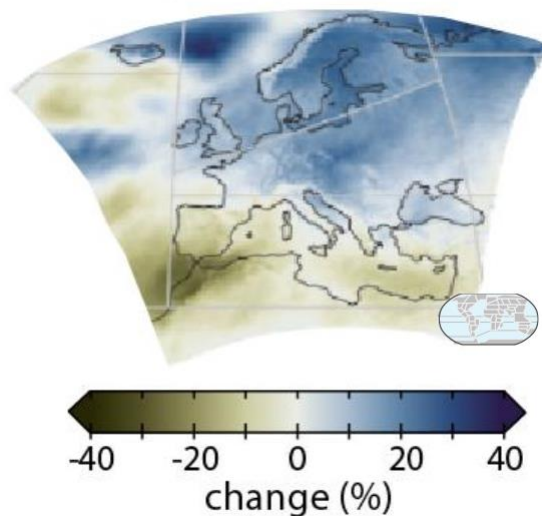
FIGURA 1.8 | Variazioni percentuali attese dell'indicatore di siccità SPI-6 per uno scenario di aumento della temperatura media globale di 2^{\circ}\text{C} .
