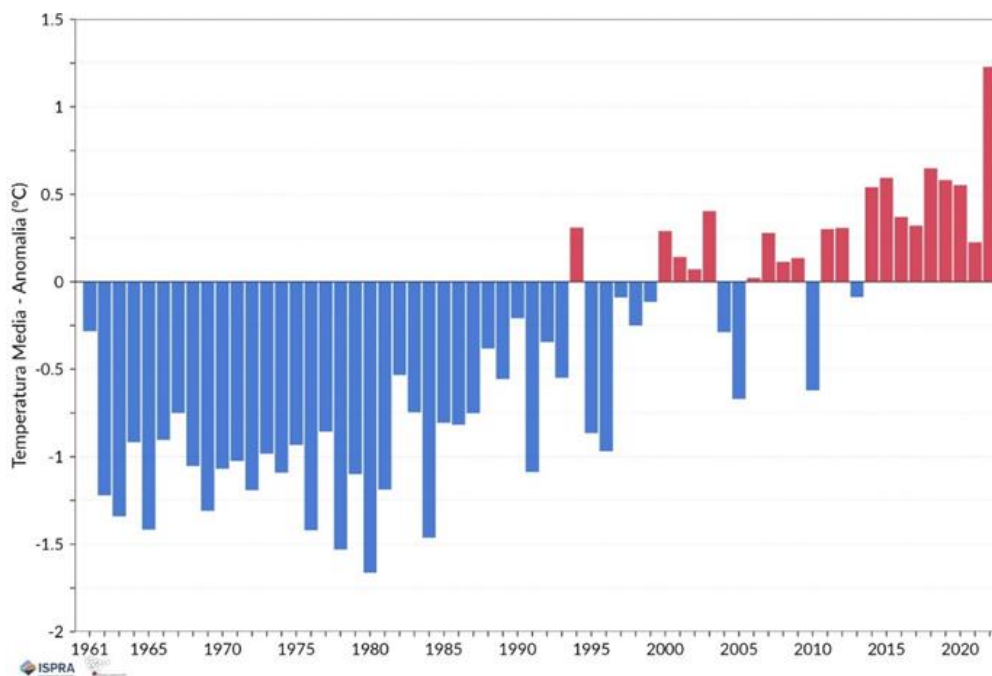
FIGURA 2.1 | Serie delle anomalie medie in Italia della temperatura media rispetto alla media climatologica 1991-2020, dal 1961 al 2022.
